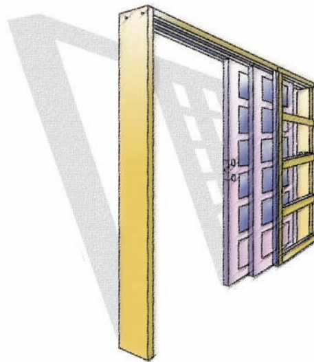
2-FLØYA SKYVEDØRSKARM med begge dørblad skjult i vegg på samme side. Type 2 : 60 TILPASSA FOR 148mm STENDER
