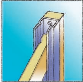
Kraftig støtteskinne i stål med patentert låsesystem for grindfjøl
