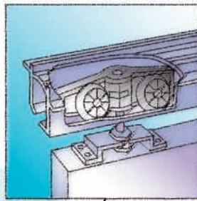
Lett rullande bogghjul med festeplate på dør
