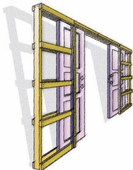
2-FLØYA SKYVEDØRSKARM
