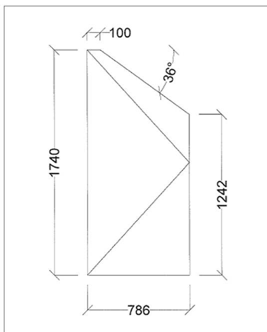
Døme på venstrehengsla dør med utvendige karmmål
