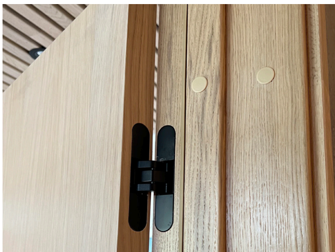
Karm med listefri løysing og skjulte hengsler. Foto: Bygg1
