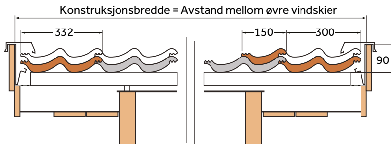
Figur 20: Konstruksjonsbredde uten bruk av gavlstien for Zanda betongtakstein
