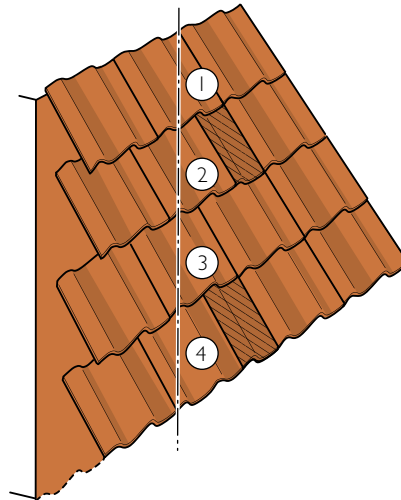
Figur 10: Forskyv kappelinjen til den samme vinkelen, slik at steinen ikke blir mindre enn halv.
