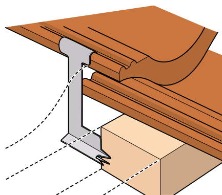
Figur 7: Feste med Stormklips 70
