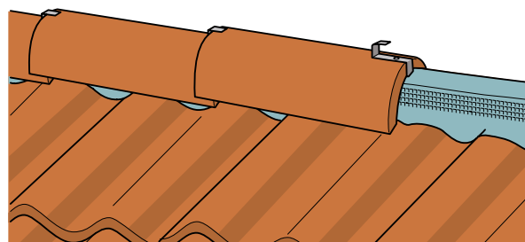
Figur 15: Feste møne- og valmstein med klips
