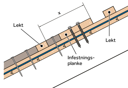
Figur 33: Montering av snøfanger
