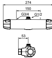
FMM 82113500 FMM 82118100
