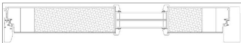
Thermokonstruksjon, U-verdi 0,57-0,98. Dørblad 86 mm.
