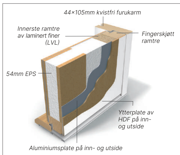
Snitt YD Forus
