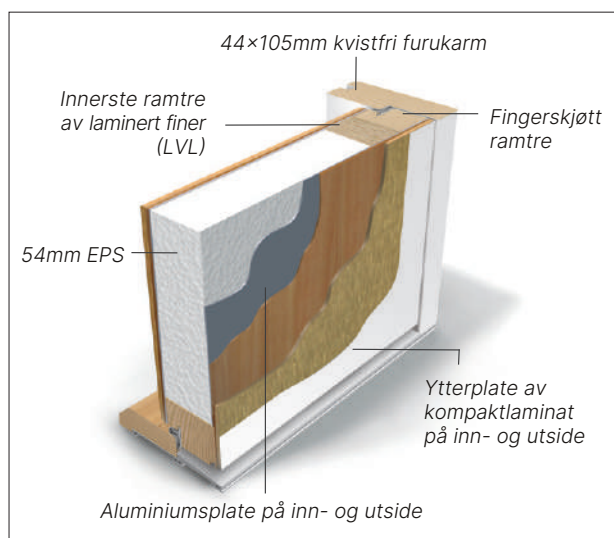
Snitt YD STD med kompaktlaminat
