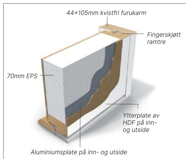
Snitt ISO
