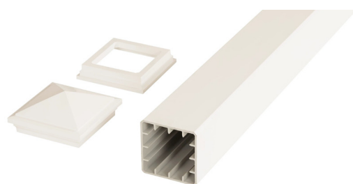
AVSLUTNINGSTOLPE M/ HATT OG LIST H 120 X B 120 x L 1000 MM
