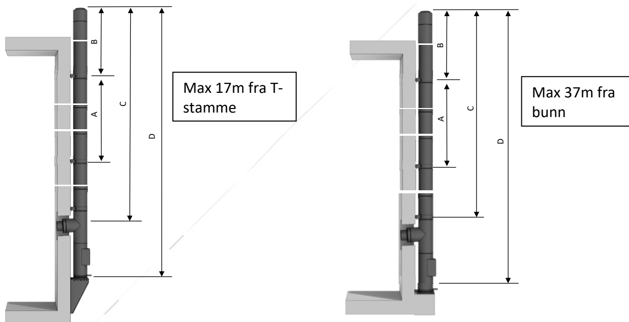
Fig. 1: Konstruksjonshøyder
