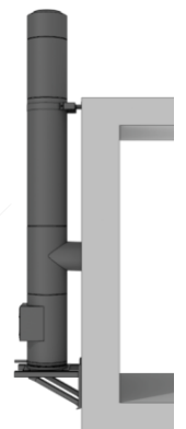
Fig. 20: Oppstilling med bunnplate med kondensatavløp og veggstøtte “vange pekende nedover ”
