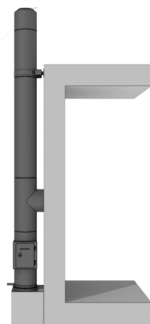
Fig. 15: Oppstilling med bunnplate for sokkelmontering
