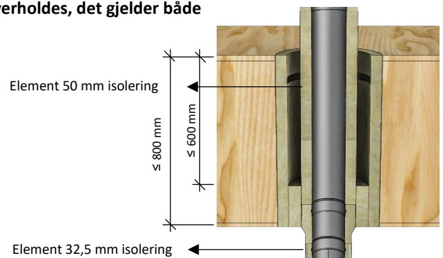
Fig. 6: Installasjon av "isolasjonsskjold" som takgjennomføring
