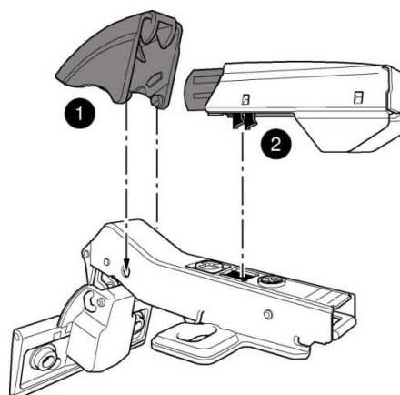
Bild på montering dämpare till 60x60-skåp
