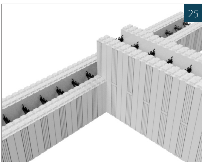
Fig. 25: I neste skift fjernes 350 mm slik at blokken kan settes inn på vangen og man får forband med skiftet under. Fra annet skift og oppover anbefales å fjerne 50 mm fra annethvert skift, slik at skruefestene i Thermomuren passer over hverandre.
