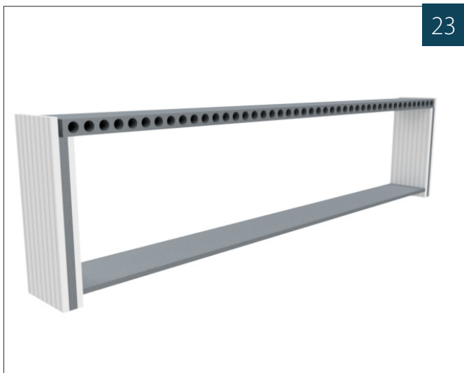
Fig. 23: Ved bruk av Thermomur® 350 kan yttervegger mot terreng utføres slik at de er støttet og innspent mot etasjeskiller i betong i overkant, og fastholdt i fundament i bunnen, uten behov for støttevegger ved utvendig oppfyllingshøyde på maks. 2,5 m.
