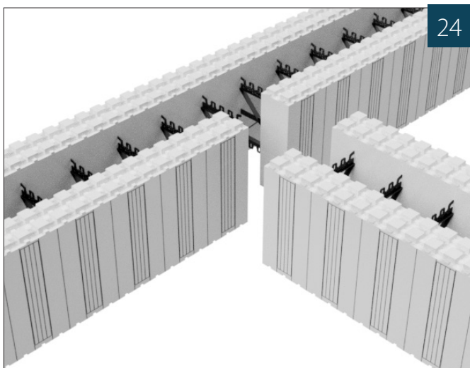
Fig. 24: I første skift: Skjær et 150 mm snitt i Thermomur®-blokkens vange slik at betongen får kontakt hele veien gjennom.
