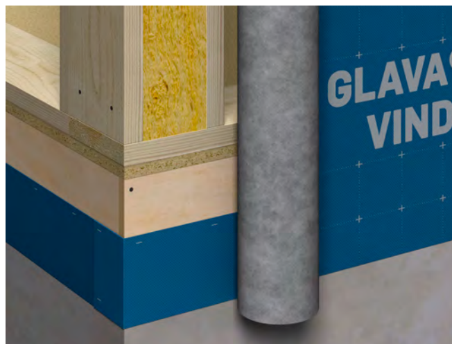
Fig. 28 Innfestet svillemembran før montering av vindspærre
