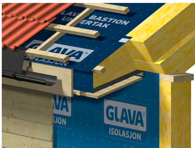
Fig. 14 Prinsipp ved utstikkende sperrer
