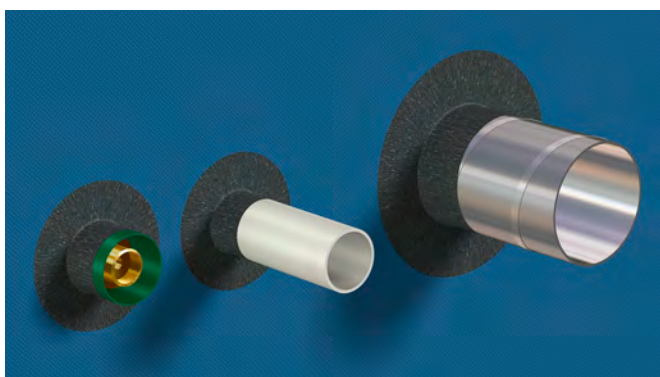
Fig. 39 Tetting av div. gjennomføringer med Glava Tettlett
