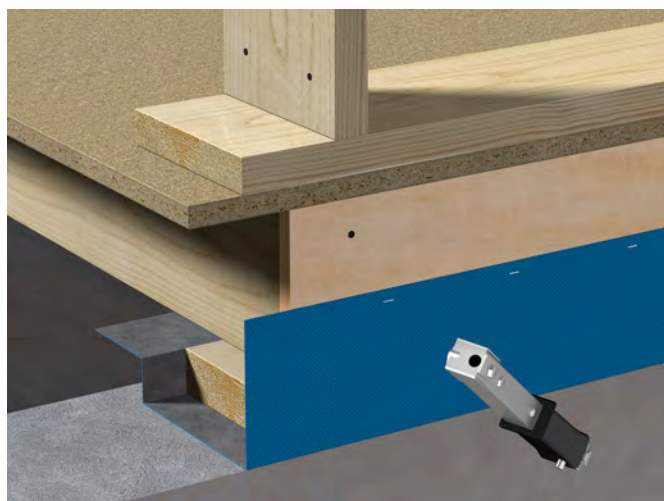
Fig. 24 Svillemembran med to lepper
