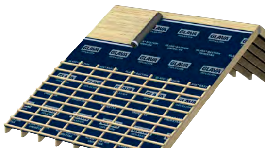
Fig. 3 viser Bastion på taktro av rupanel
