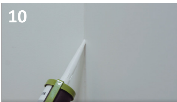
10 HUNTONIT AKRYLMASSE ANBEFALES TIL INNVEINDIGE HJØRNER.
