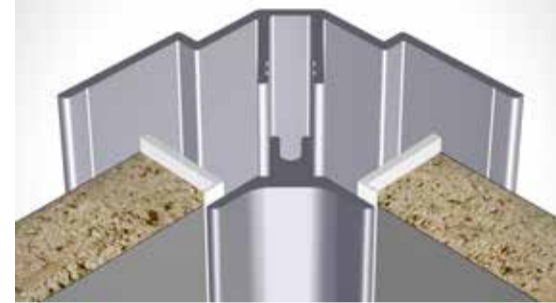
Fig. 4 Skjøtelist ved ekspansjonsfug/ Moulding for expansion clearance
