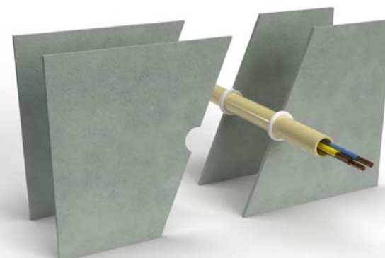
Fibercement med PVC-rør og kabler: FP310 INTUMESCENT ACOUSTIC ACRYLIC
