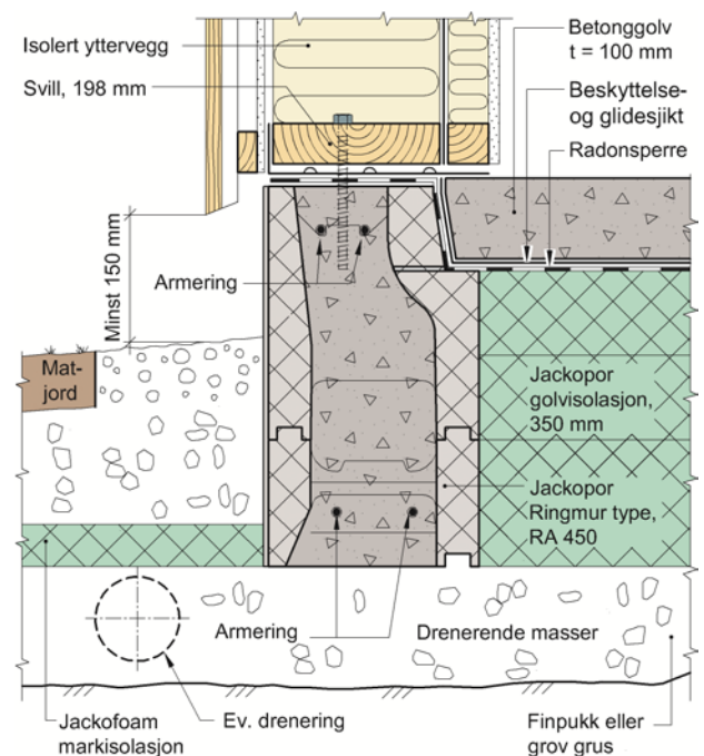
Fig. 3 Eksempel på bruk av Jackopor Ringmur type RA 450
