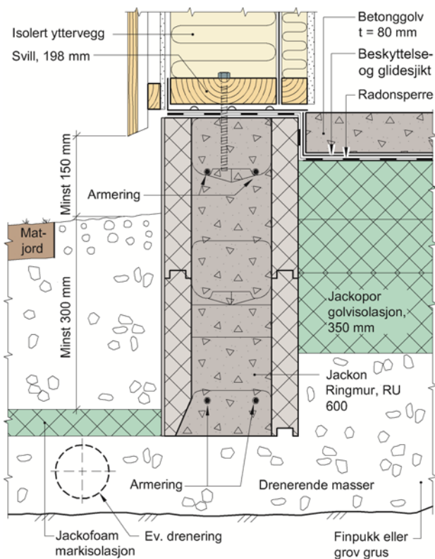
Fig. 4 Eksempel på bruk av Jackopor Ringmur type RU 600
